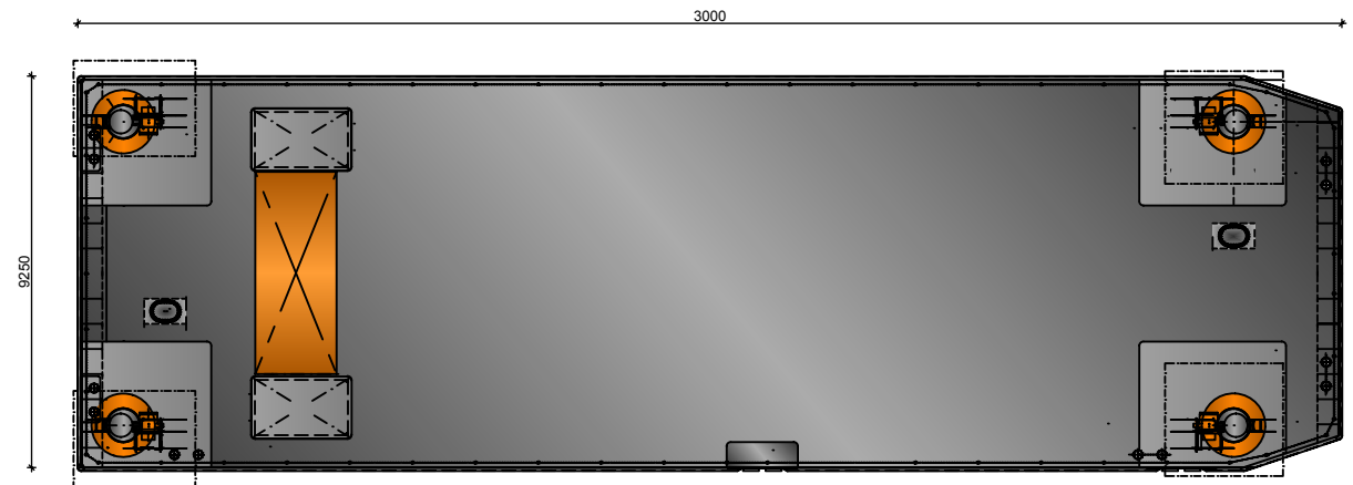
Draufsicht
